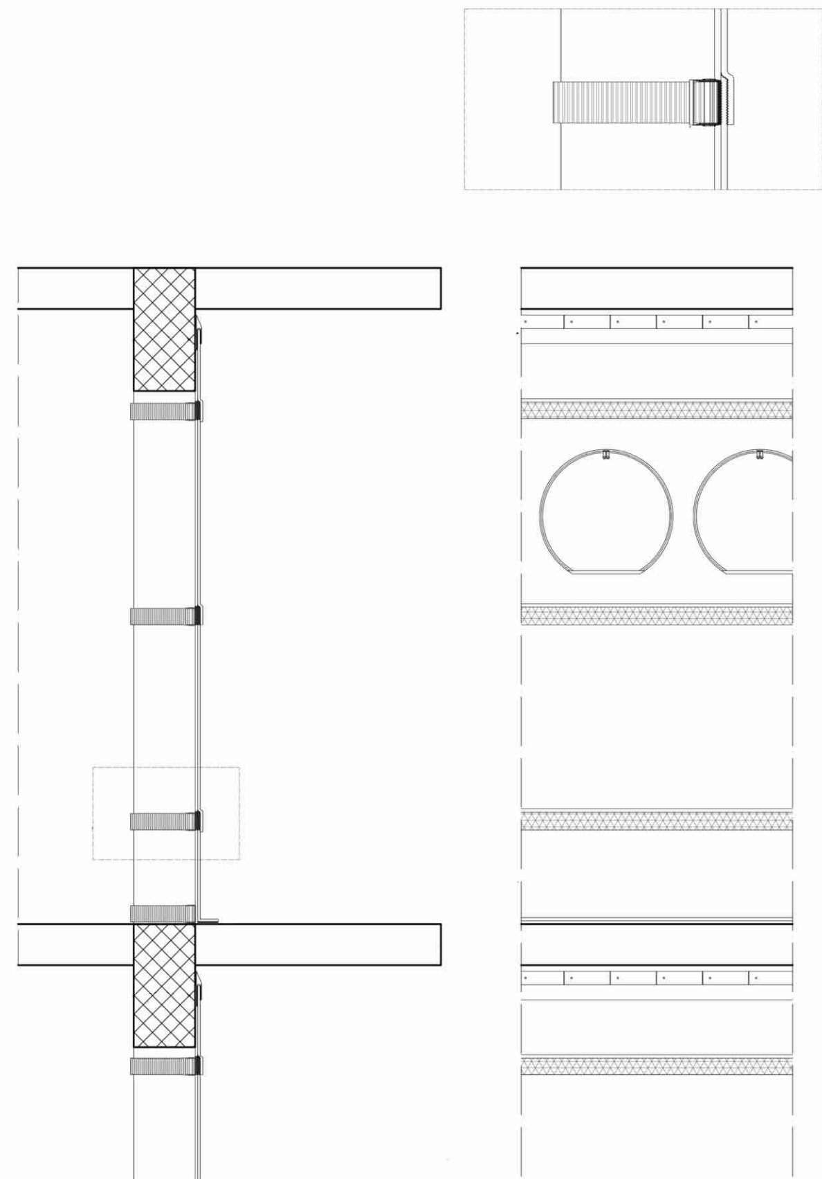
sezione e prospetto del sistema involucro
