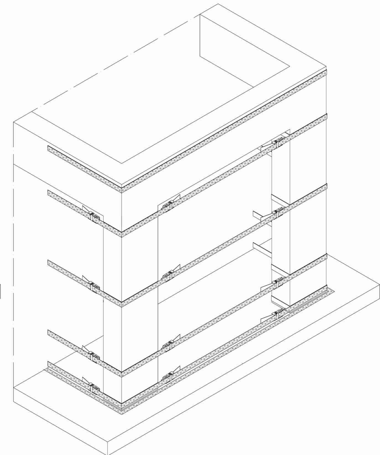
Struttura con cinghie orizzontali
